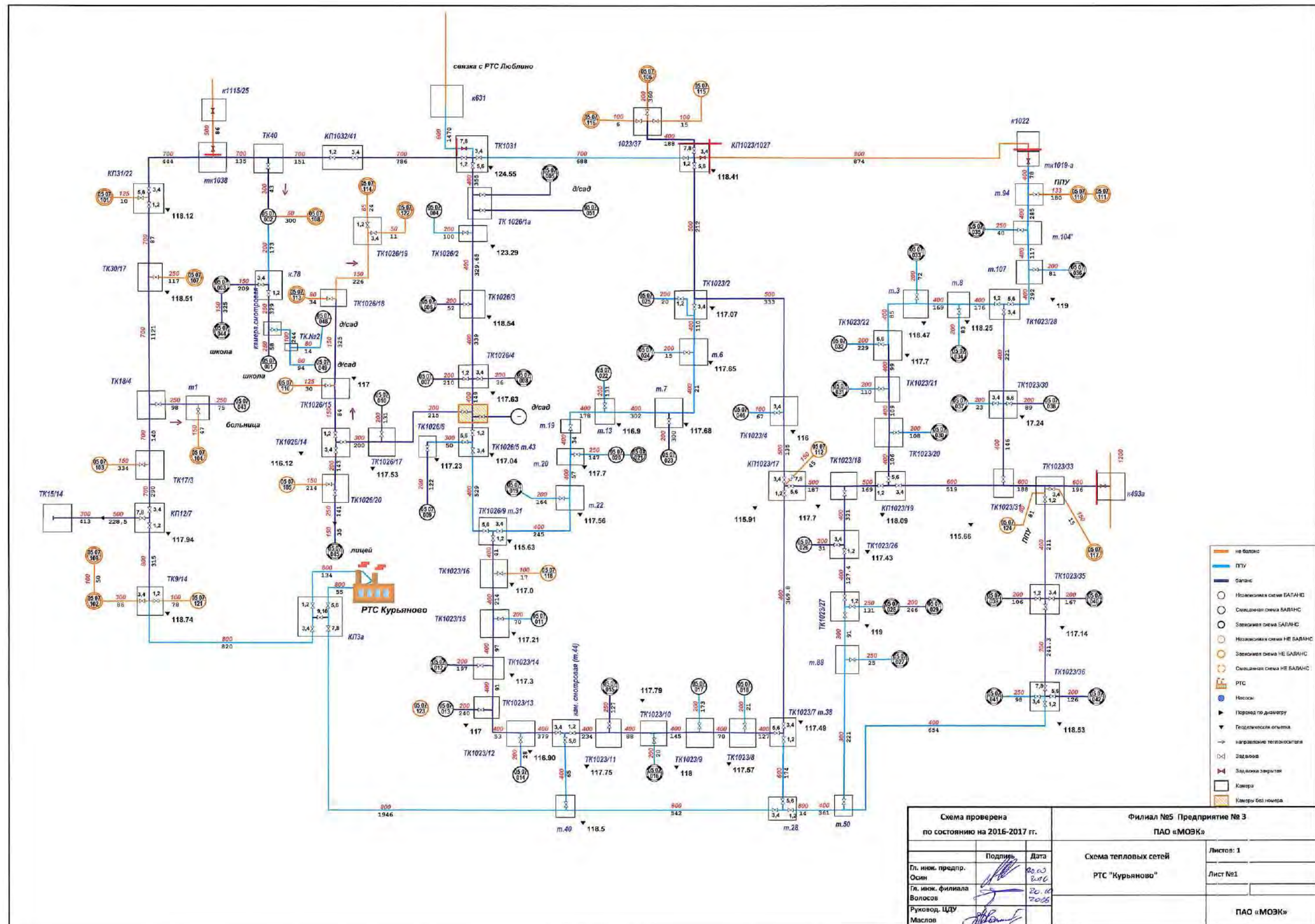
Рисунок А.14.2 - Схема тепловых сетей от РТЭС «Курьяново»
