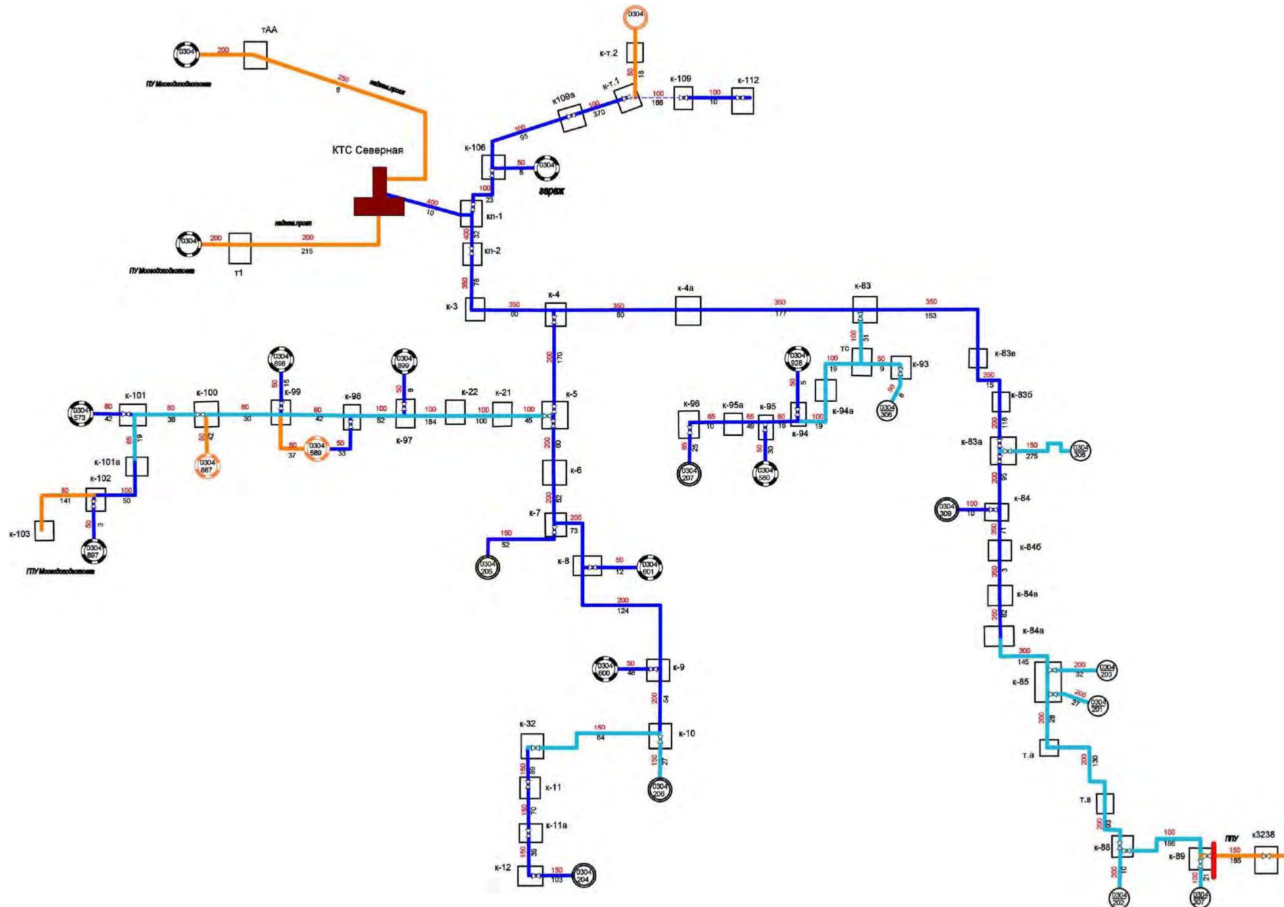
Рисунок А.15.4 - Схема тепловых сетей от КТС «Северная»
