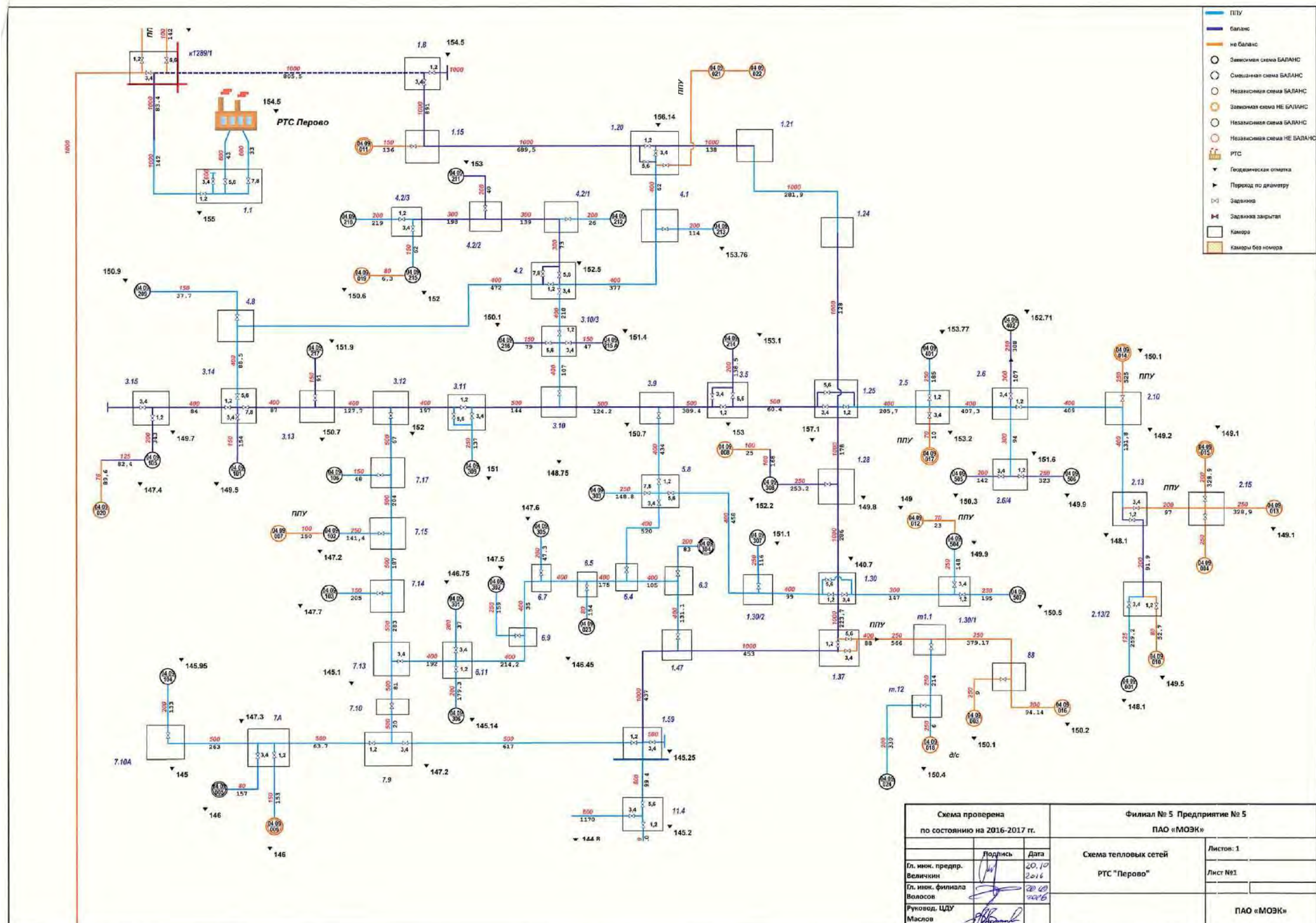
Рисунок А.14.14 - Схема тепловых сетей от РТС «Перово»
