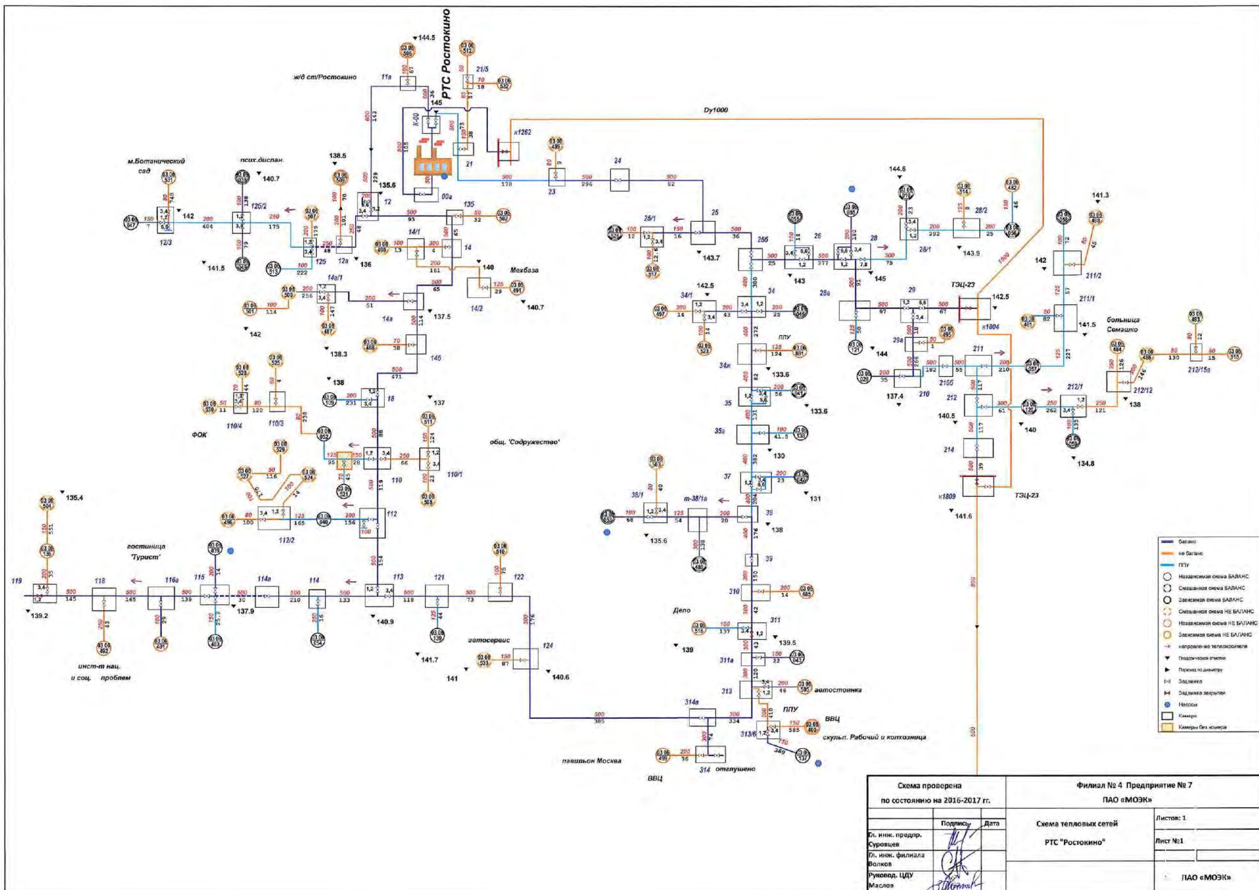
Рисунок А.14.6 - Схема тепловых сетей от РТС «Ростокино»
