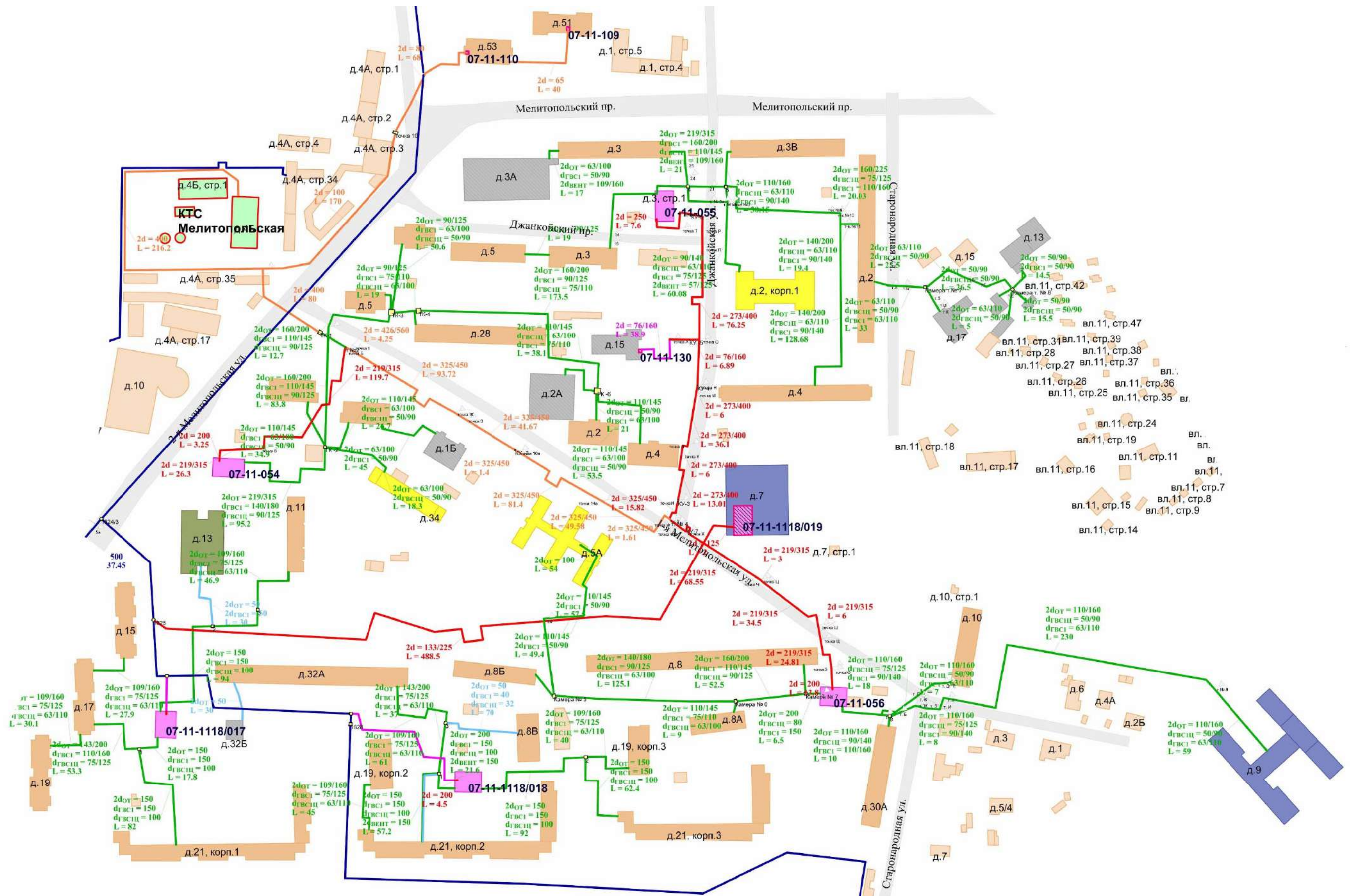
Рисунок А.15.6 - Схема тепловых сетей от КТС «Мелитопольская»
