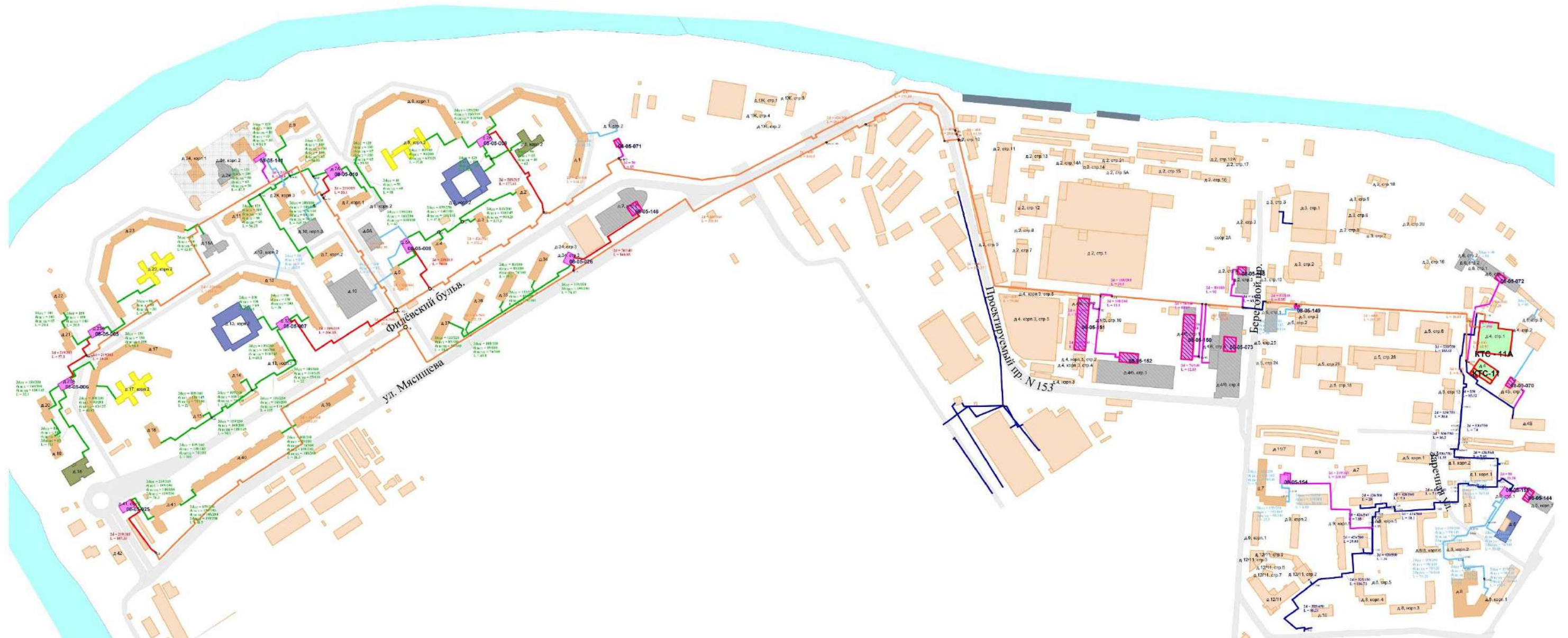
Рисунок А.15.1 - Схема тепловых сетей от КТС-11 и КТС-11А
