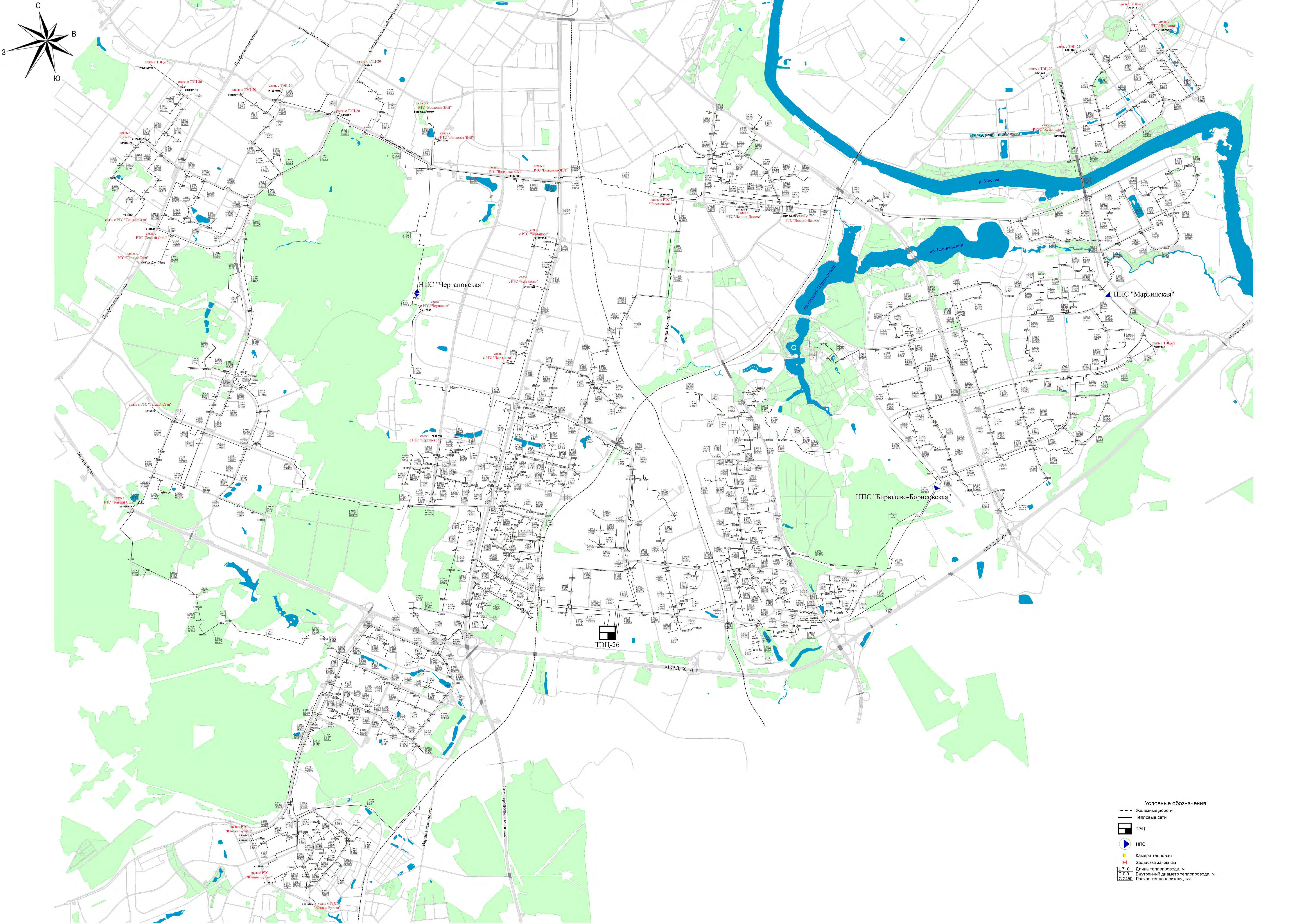
Расчетная схема тепловых сетей от ТЭЦ-26
