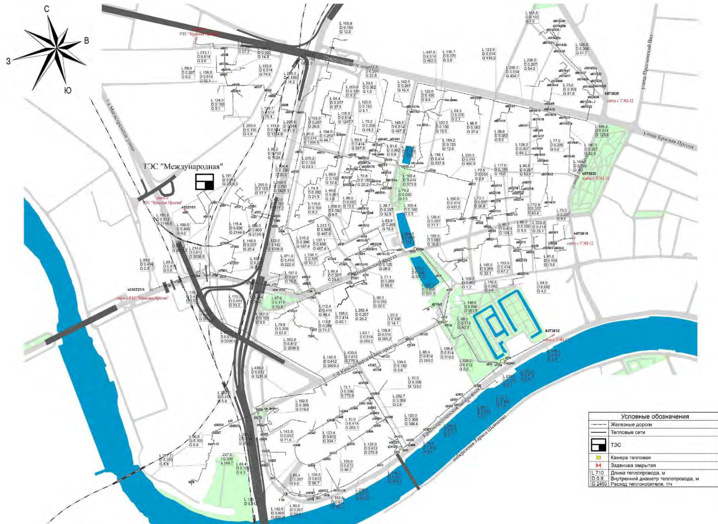
Рисунок А.14.4 - Схема тепловых сетей от ТЭС «Международная»
